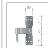
Kreuzband Standard
