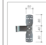
Kreuzband Standard
