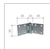
Scharnier für Doppelflügel
