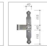
Mittelband Rustikal
