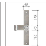
Mittelband Standard
