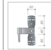
Kreuzband Standard
