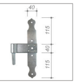
Mittelband Rustikal
