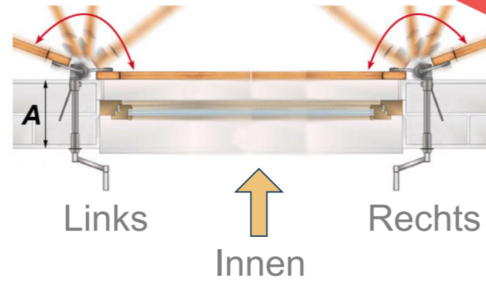
2F/1R1L Zweiflügelig Fenster / 1 Einfachflügel links, 1 Einfachflügel rechts
