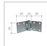
Scharnier für Doppelflügel
