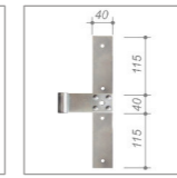
Mittelband Standard
