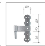
Kreuzband Rustikal
