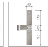
Mittelband Standard
