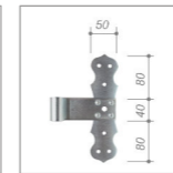
Kreuzband Rustikal
