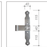
Mittelband Rustikal
