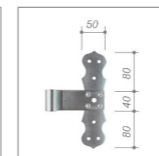
Kreuzband Rustikal
