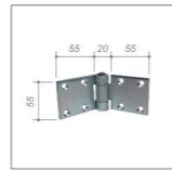
Scharnier für Doppelflügel
